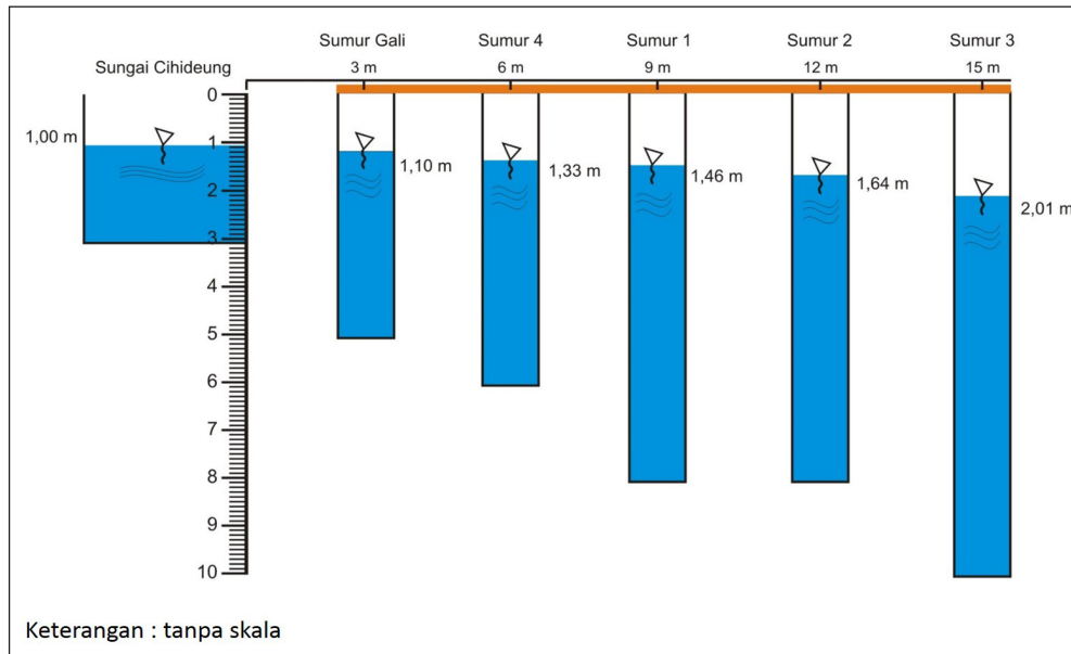
Gambar 2. Tata Letak Sumur di Lokasi Penelitian.
