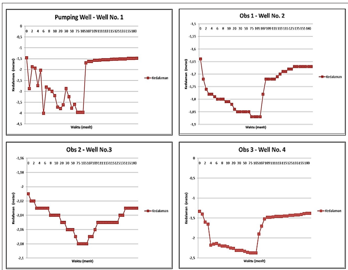
Gambar 2. Kurva Penurunan dan Imbuhan Muka Air Tanah pada Sumur Uji ( Pumping Well ) dan Sumur Pengamatan (Obs 1, Obs 2, Obs 3).
