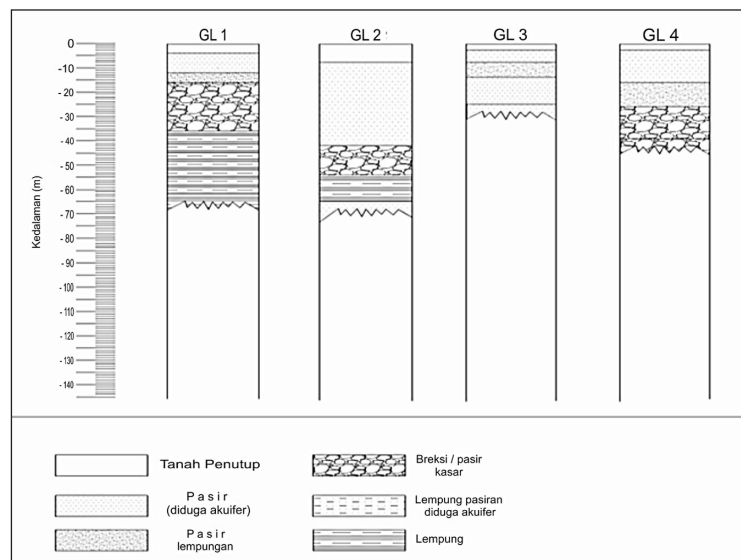
Gambar 1. Model log bor hasil penafsiran data geolistrik.
